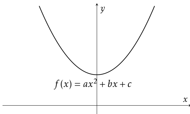
Figur 2: Andengradspolynomium.
