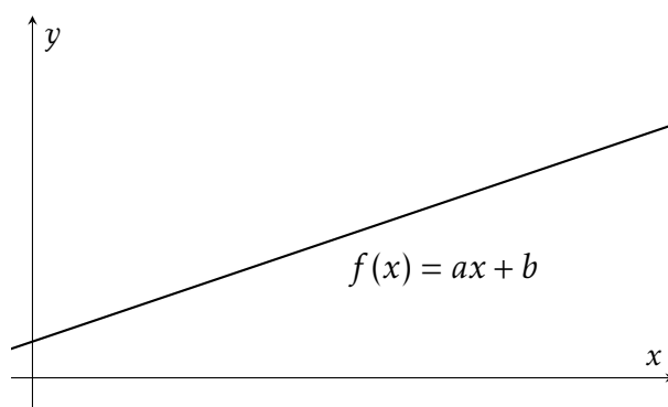
Figur 1: Et førstegradspolynomium.
