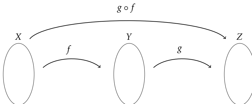
Figur 1: En sammensat funktion
